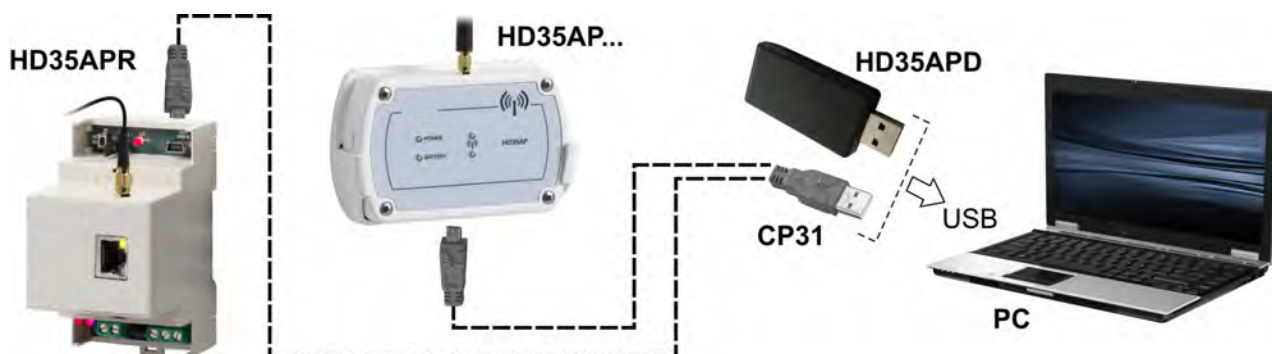
Fig. 6.4.1: connexion USB
