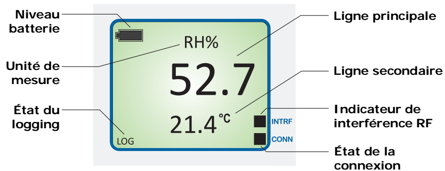
Fig. 10.5.1: LCD custom
