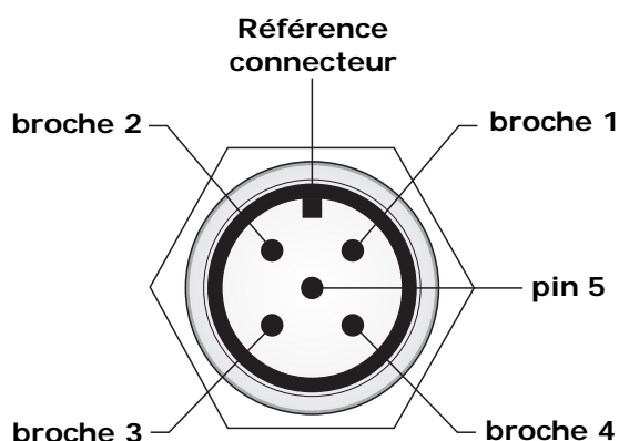
Fig. 9.9.1: vue extérieur du connecteur M12 de l'instrument
