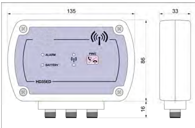
HD35ED... versions avec connecteurs M12
