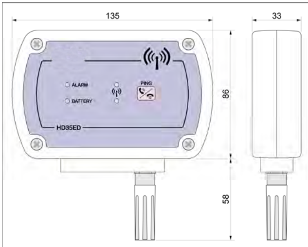
HD35ED... versions avec sonde HR/T fixe
