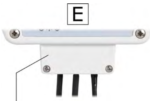
Entrées à bornes protégées par un couvercle (voir par. 8.5 pour la position des bornes)
