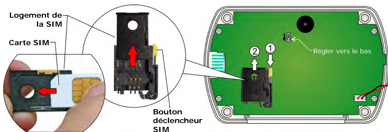
Fig. 6.9.1: insertion de la carte SIM dans HD35APG et HD35AP3G
